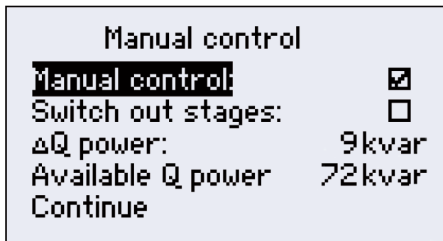
图 36 开启手动控制
