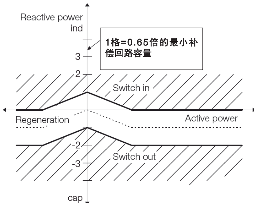
图 50 目标功率因数= - 0.95，限值= - 1.0，平移=0时的控制曲线
