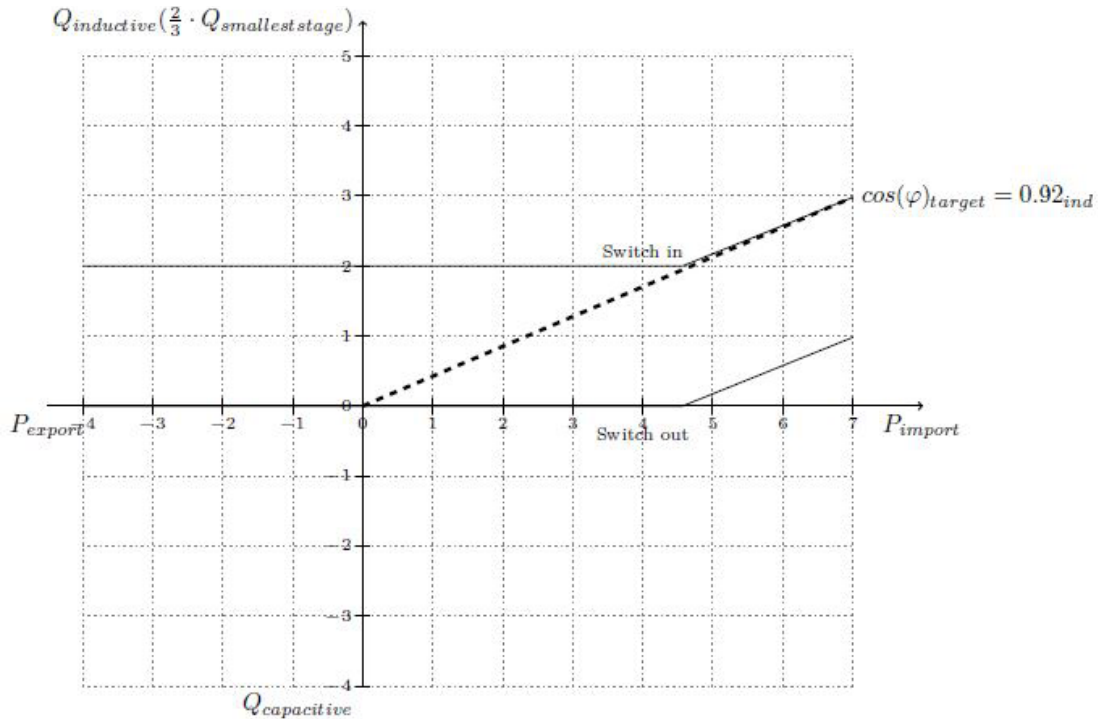
Profile 1 目标功率因数=0.92, 限值=1.0, 平移值=-1.0时的控制曲线图
