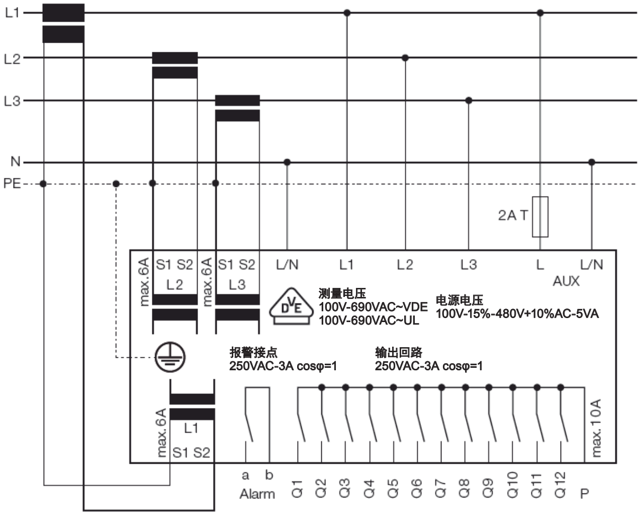
图 6 PQC 1204803-XX 接线原理图
