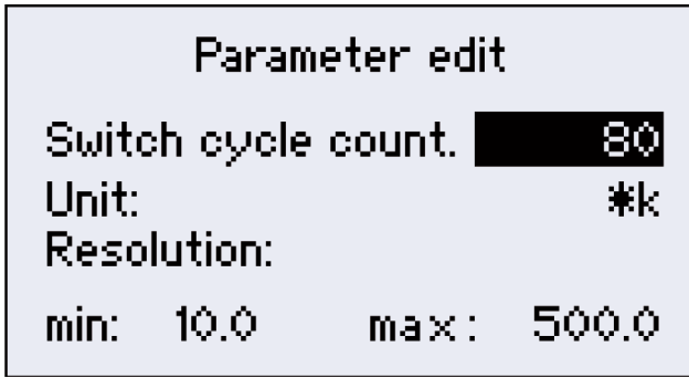
图 56 改变循环投切计数的范围
