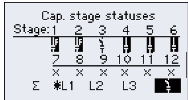
图 31 补偿回路状态 (三相, 12路)
