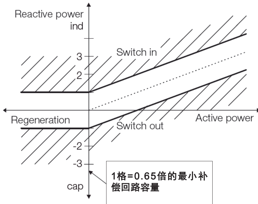
图 45 目标功率因数=0.92, 限值=0, 平移值=0时的控制曲线图
