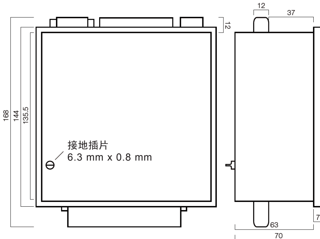
图 1 PQC 尺寸图 (mm)
