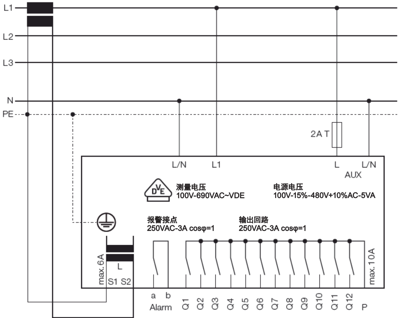
图 5 PQC 1204801-XX 接线原理图
