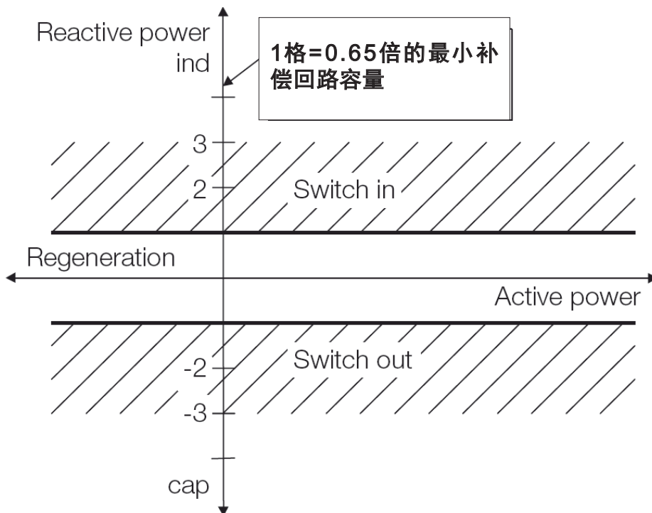
图 44 目标功率因数=1, 限值=0, 平移值=0时的控制曲线图
