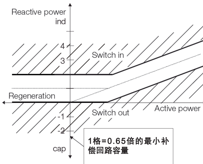
图 48 目标功率因数=0.92, 限值=+1.0时的控制曲线
