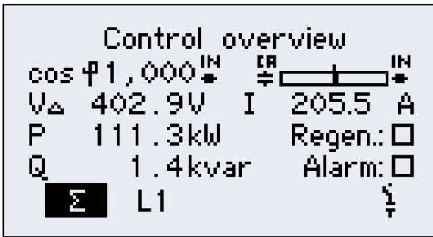
图 28 PQC 概览 L1 (单相)
