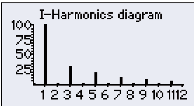
图 77 电流谐波图, Y轴100%
