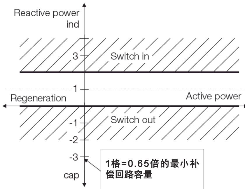
图 46 当参数设置为目标功率因数=1, 限值=0, 平移值=+1.0时的控制响应图
