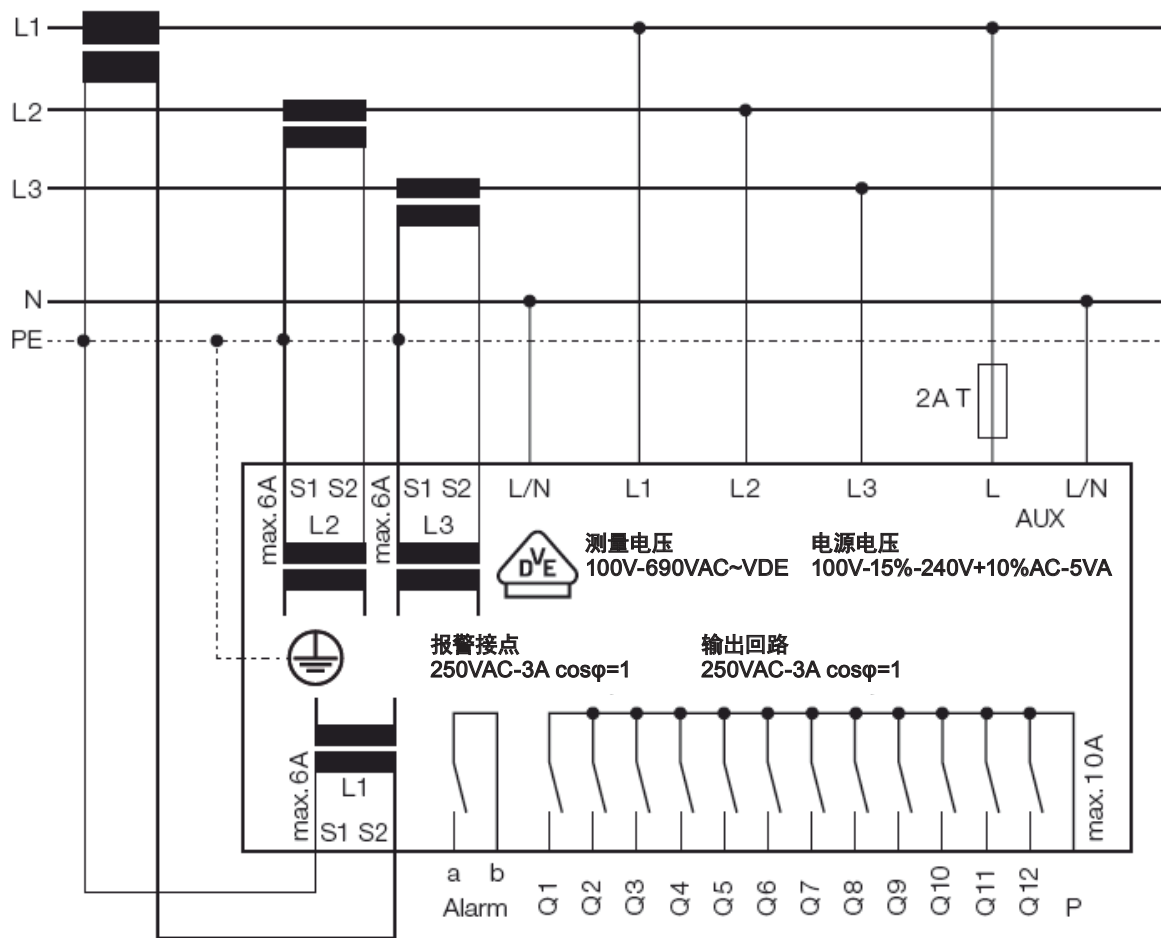
图 3 PQC 1202403-XX 接线原理图
