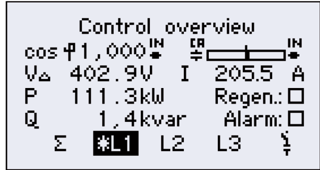
图 29 PQC 概览 L1 (三相)
