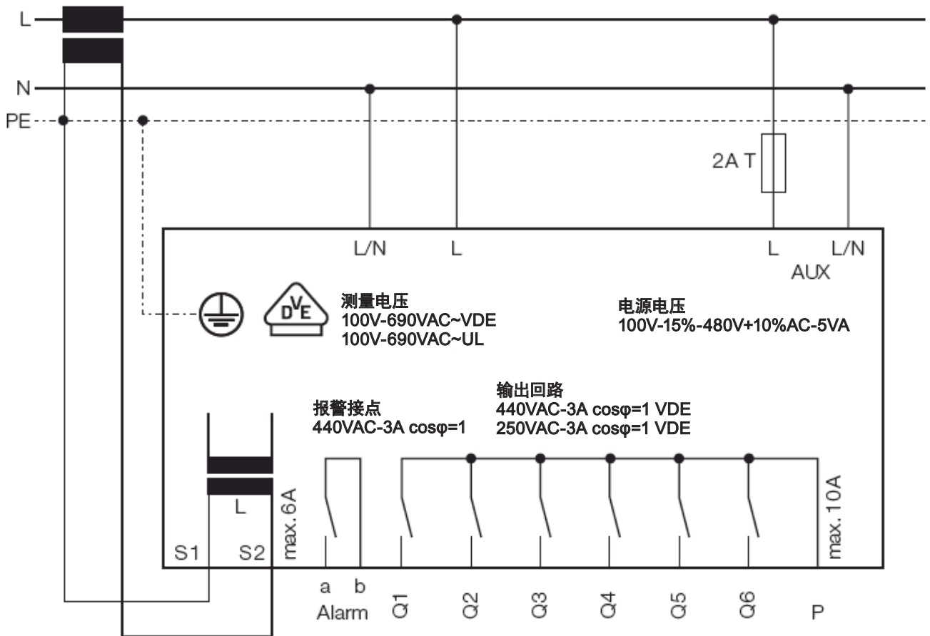
图 7 PQC 0614801-XX 接线原理图
