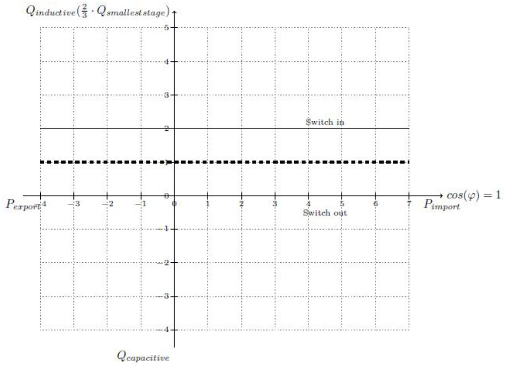
Profile 3 目标功率因数=1, 限值=0, 平移值=1.0时的控制曲线图
