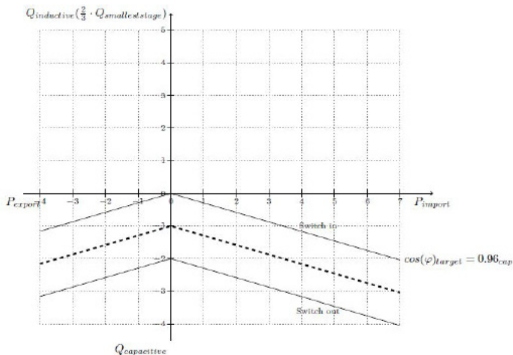
Profile 5 目标功率因数=0.96, 限值=0, 平移值=-1.0时的控制曲线图
