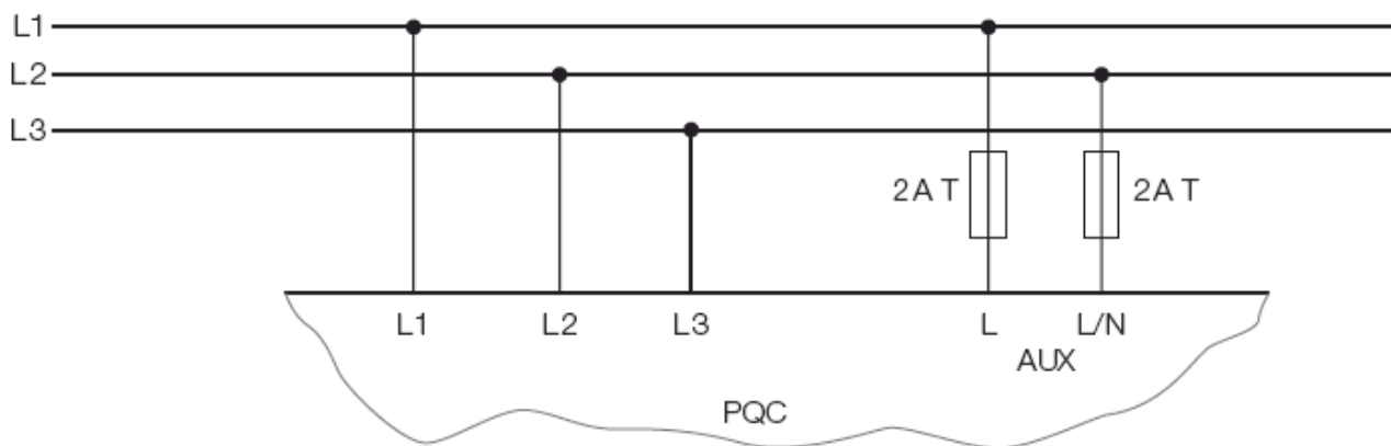
图 8 PQC在400/415V无零线电网的部分接线原理图
