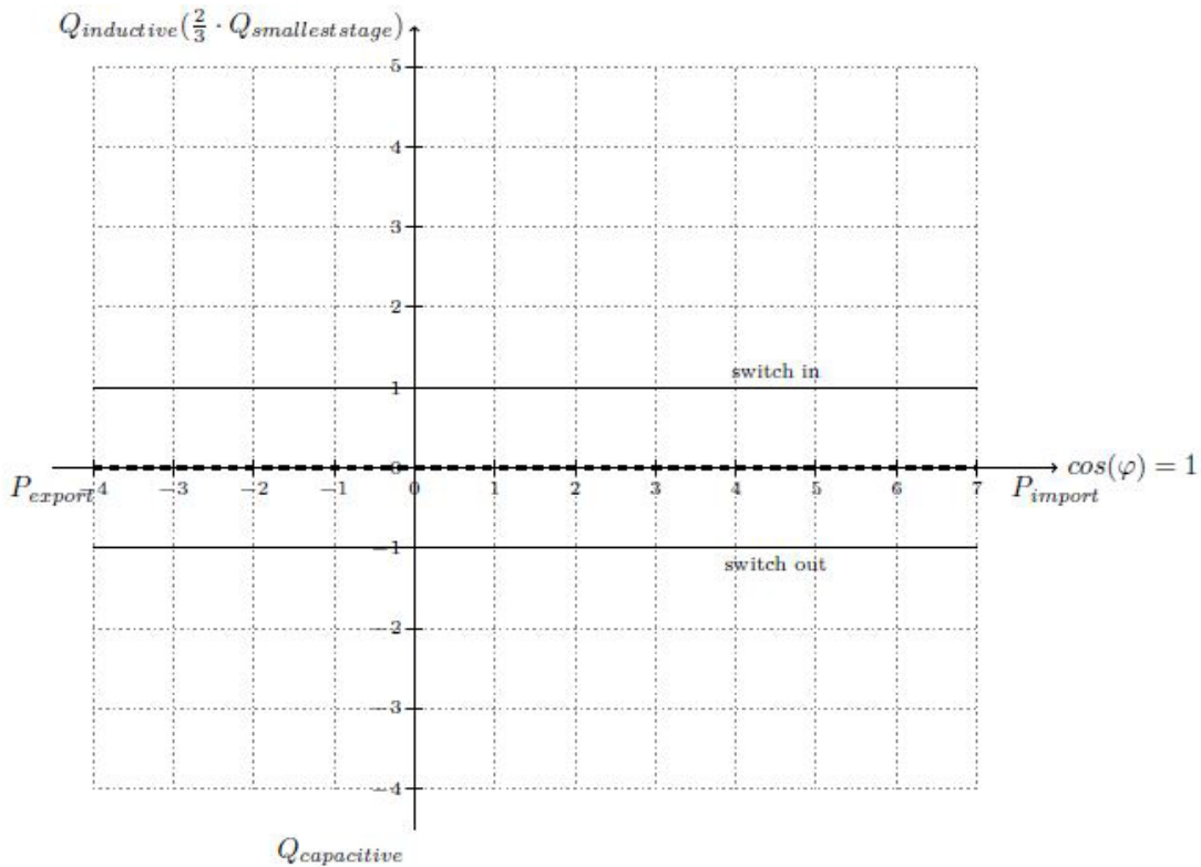
Profile 2 目标功率因数=1, 限值=0, 平移值=0时的控制曲线图
