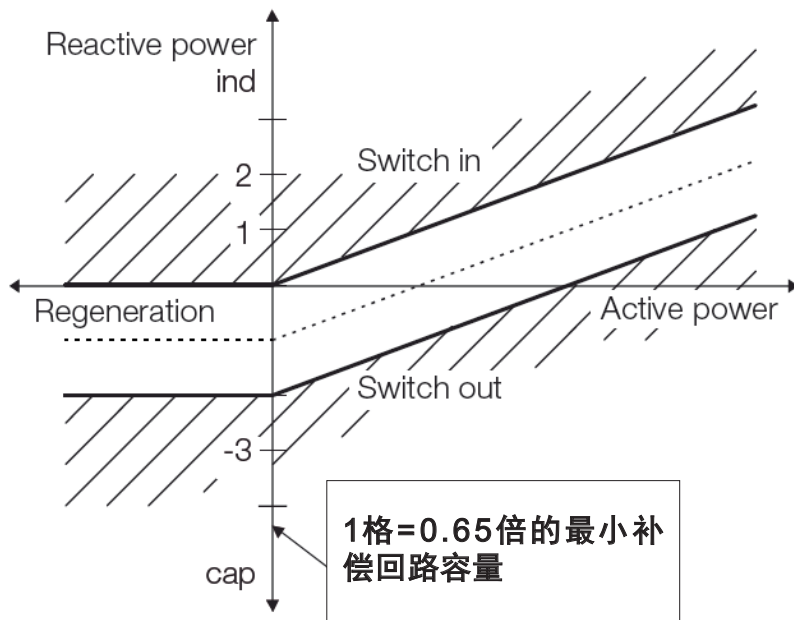
图 47 当参数设置为目标功率因数=0.92, 限值=OFF, 平移值=-1.0时的控制响应图
