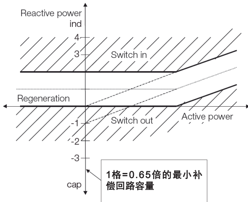
图 49 目标功率因数=0.92，限值=+1.0，平移=-1.0时的控制曲线
