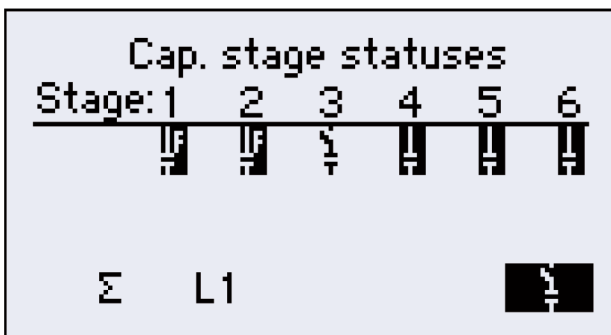
图 30 补偿回路状态 (单相, 6路)
