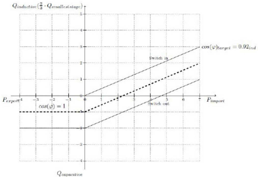
Profile 4 目标功率因数=0.92, 限值=0, 平移值=-1.0时的控制曲线图
