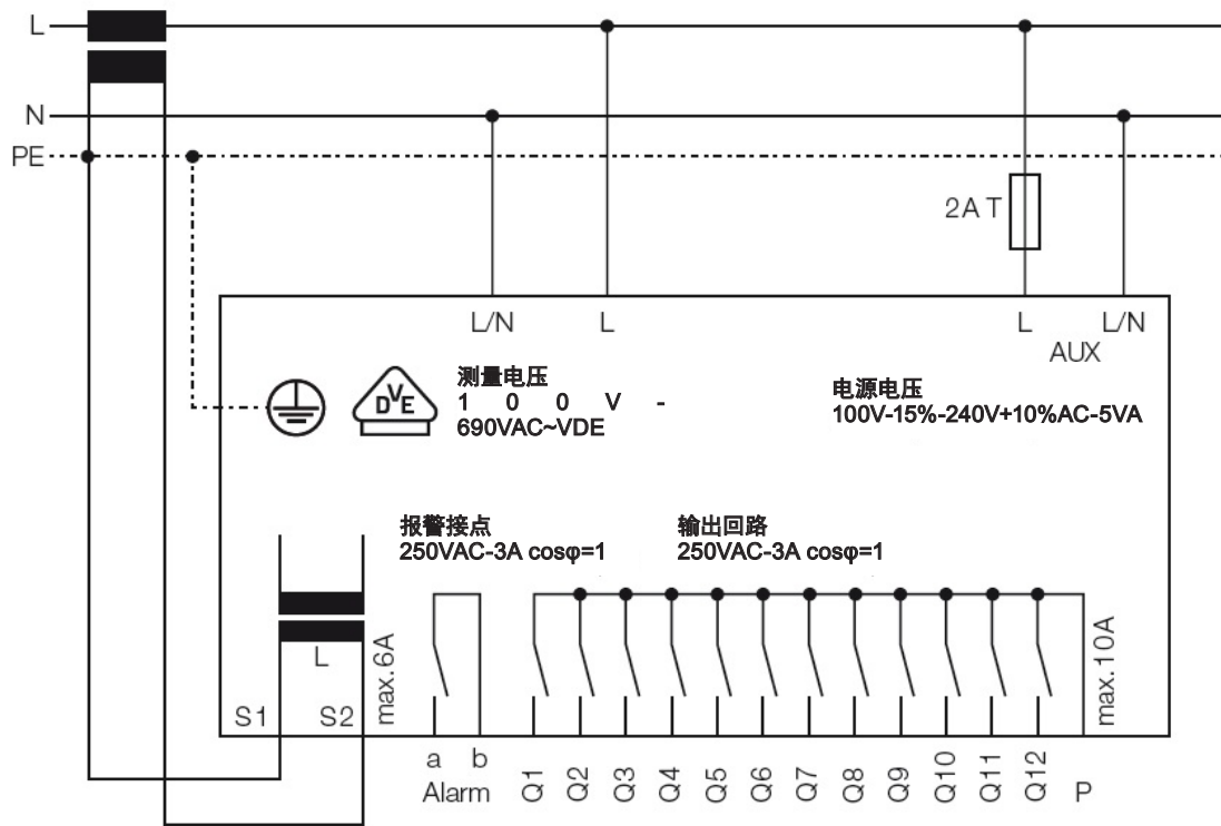
图 2 PQC 1202401-00 接线原理图
