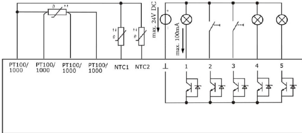
图 61 无源数字输入输出和温度传感器输入回路
