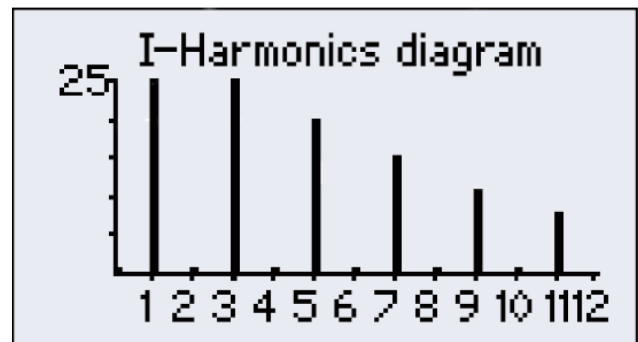
图 78 电流谐波放大, Y轴25%
