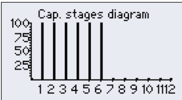
图 74 显示所有回路补偿容量为100%
